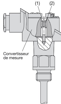
Fig. 3. Montage avec ressort d'amortissement sur un élément de mesure.
