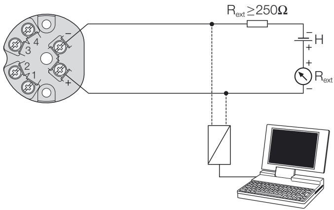
Fig. 8. Configuration d'un SINEAX VK 626 en exécution standard.
